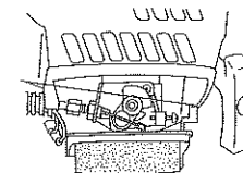
Tornillo M3 Ayustador Conecte el cable al final del ajustador Tornillo de ajuste del ralenti
