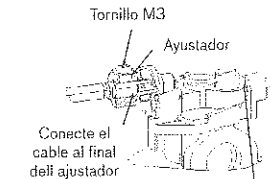
Tornillo M3 Ayustador Conecte el cable al final del ajustador Tornillo de ajuste del ralenti
