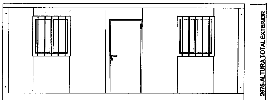
VISTA LATERAL
