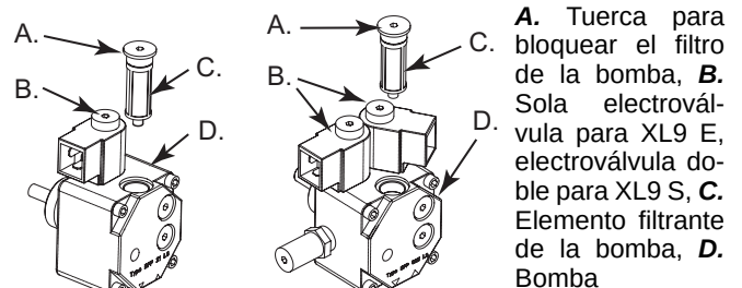
Figura 11 - Bomba del quemador XL9E y XL9 S.
