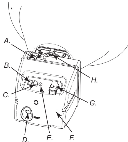
Figura 5 - Controles de la función XL9 E.
