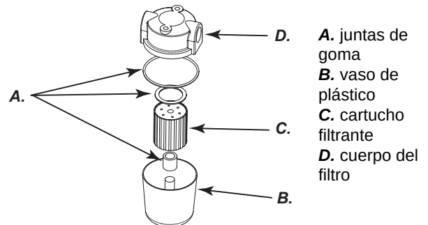
Figura 10 - Filtro de gasóleo XL9.
