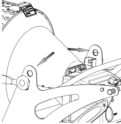
Figura 7 - Ganchos para levantar.
