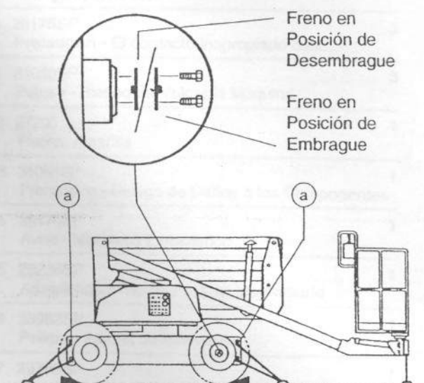
a puntos para levantar la máquina con grúa
