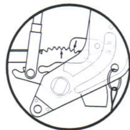
C. Demasiado flojo; ajustar los cables de freno (Sección 5.6.3)
