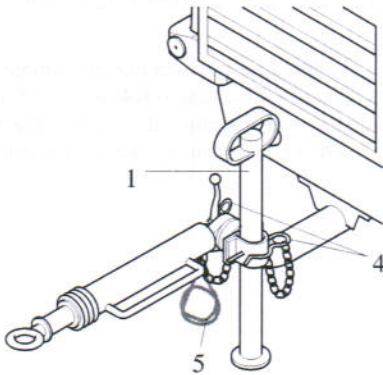
Fig. 3.1 Barra de remolque no ajustable con soporte estándar sin frenos
