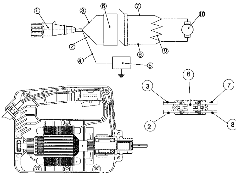
MOTOR AVMU - TRANSMISIONES Y AGUJAS
