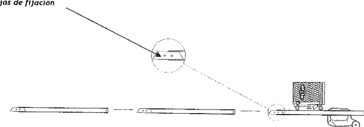
Fig.21: Montaje de los tramos
