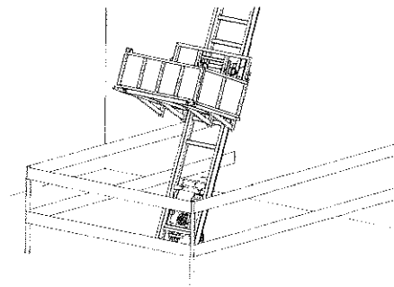
Fig. 23: Protección de la base
