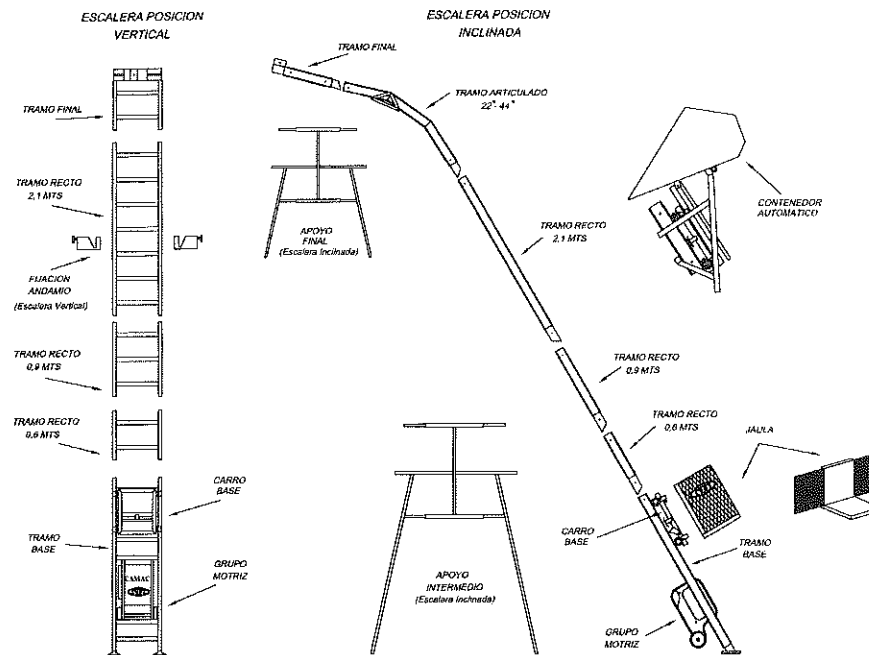
Fig. 01: Componentes Minor Escalera
