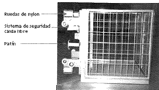
Fig. 10: Carro base
