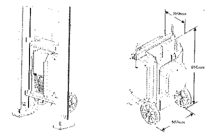
Fig.03: Grupo motriz
