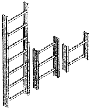
Fig.07: Tramos rectos de 2,1m, 0,9m y 0,6m
