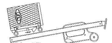
Figura 20: Montaje del carro base más la jaula monta-materiales
