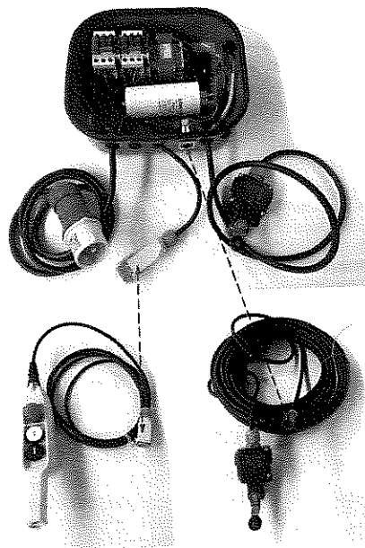
Fig. 22: Conexiones al módulo
