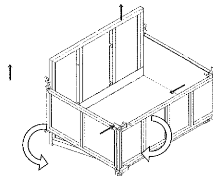
Fig. 12: Estructura jaula aluminio de 3 rampas
