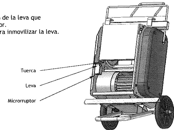
Fig.24: Zona de regulación de la leva
