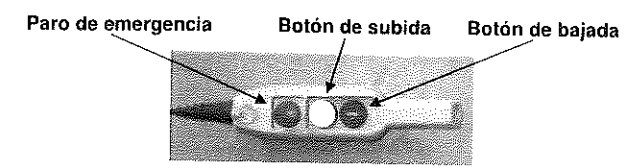
Fig.04: Botonera de mando
