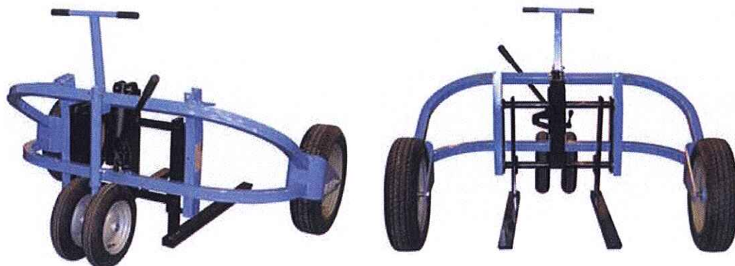
Detalle de las ruedas direccionales Detail of directional wheels Détail des roues directionnelles
