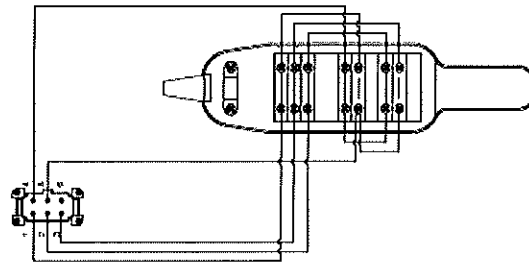
BOTONERA TELEMANDO N°2 Modelo PC-03.1
