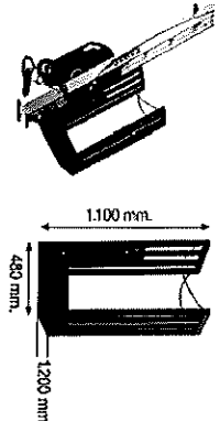
JAULA ESTANDAR
